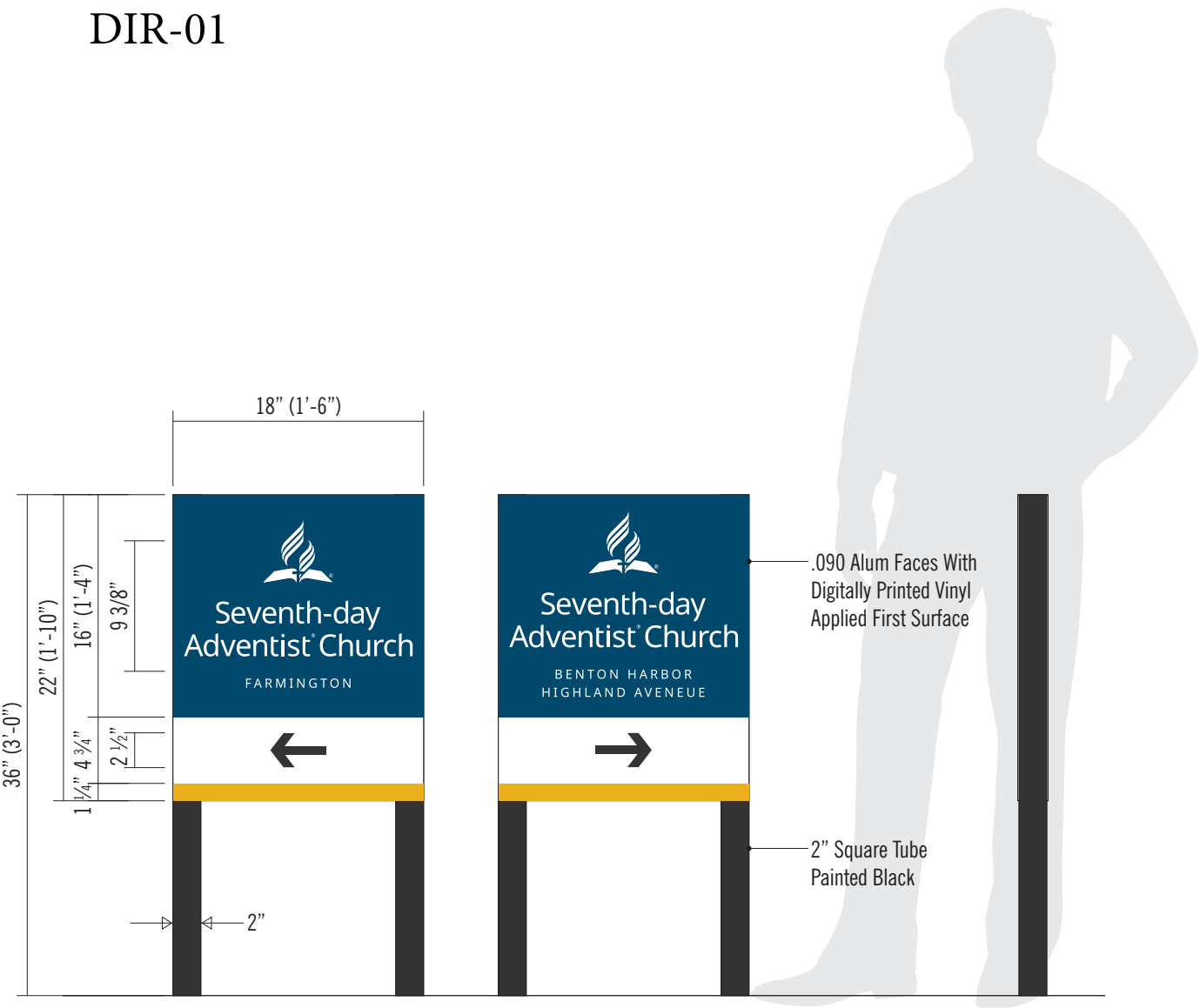
Scale: 1"=1'-0"
